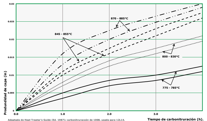
Gráfica de carbonitruración para acero AISI 12L14.
